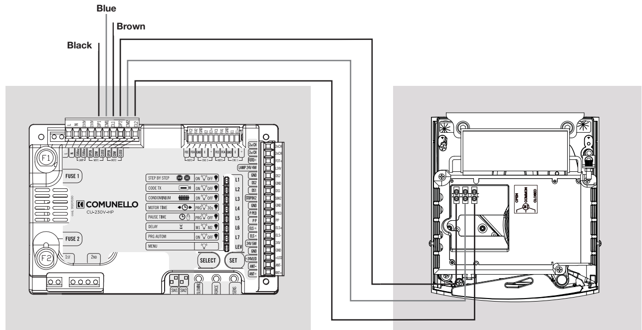
CONDOR [2/2]- schema di collegamento dei motori
